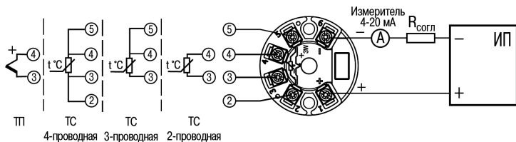
Рисунок 6.3 – Подключение прибора
